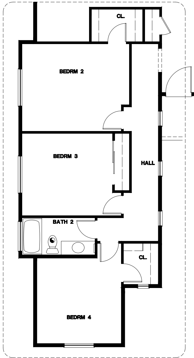
OPT. BEDRM 4
